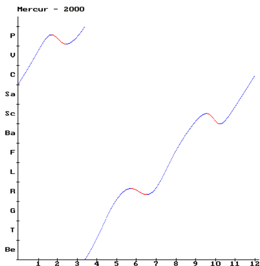
Pozițiile lui Mercur în anul 2000.
