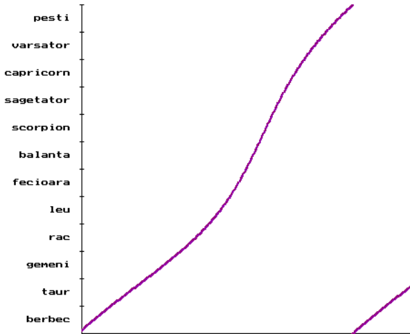
Drumul lui Pluto în 300 de ani.
