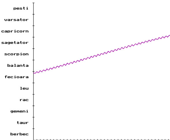
Pozițiile lui Pluto, din 1970 până în 2010.
